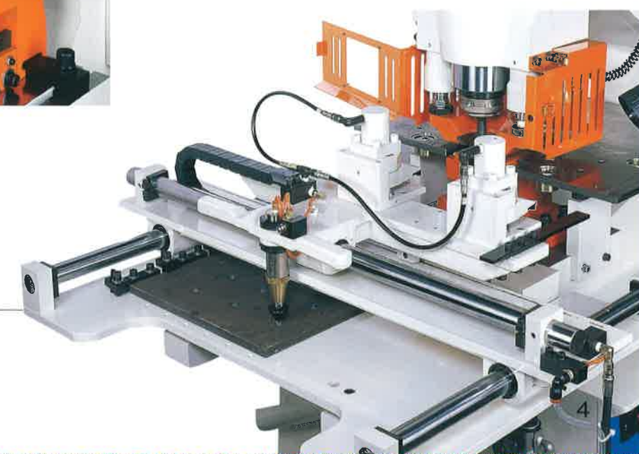
*Pliage d'angle
